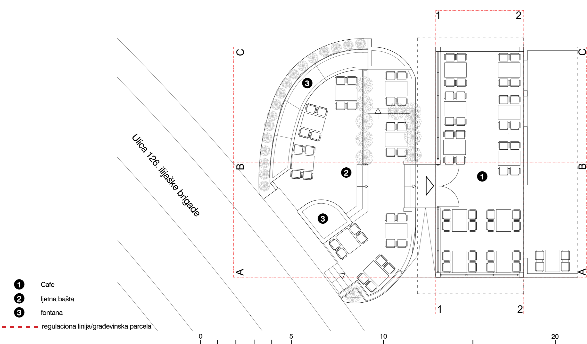
TLOCRT
