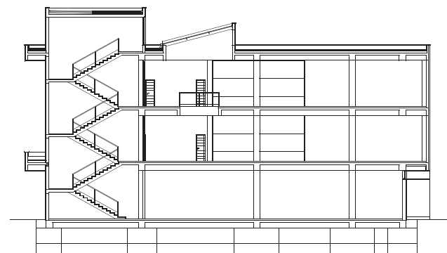
KARAKTERISTIČNI PRESJEK
