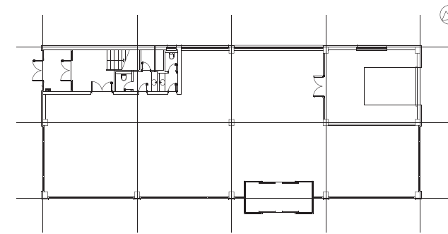
OSNOVA PRIZEMLJA
