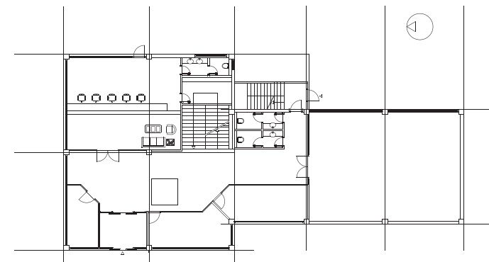
OSNOVA PRIZEMLJA
