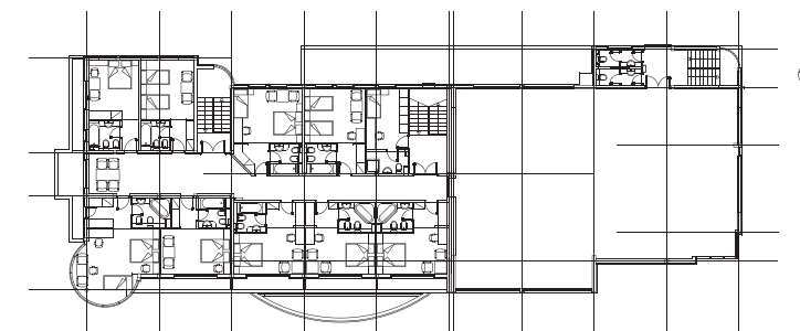
OSNOVA II KATA
