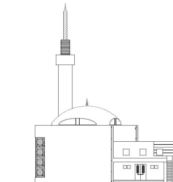
KARAKTERISTIČNA FASADA
