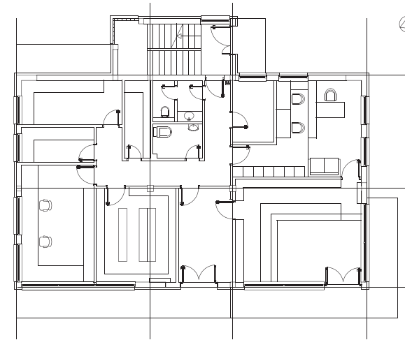
OSNOVA PRIZEMLJA
