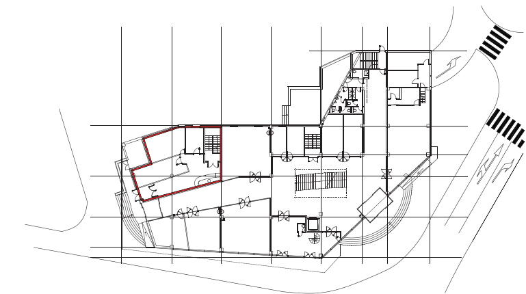
OSNOVA PRIZEMLJA
