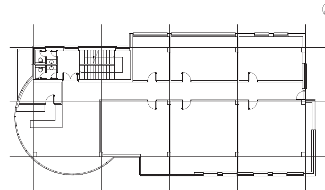
OSNOVA KATA
