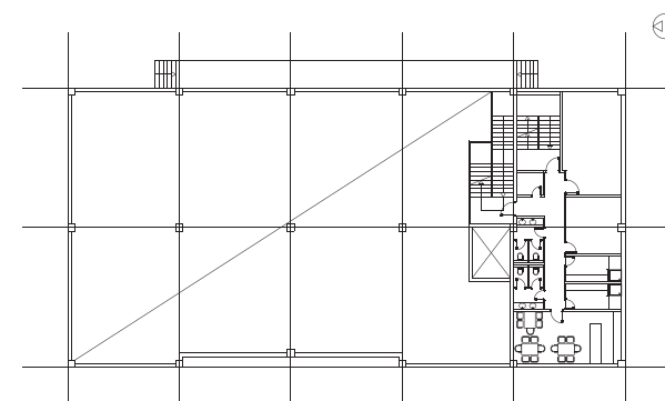
OSNOVA MEĐUETAŽE
