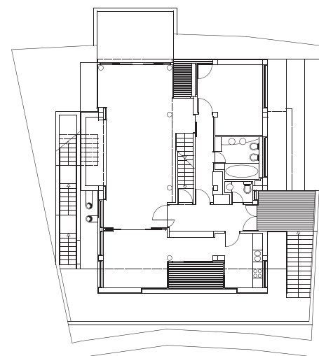
OSNOVA PRIZEMLJA
