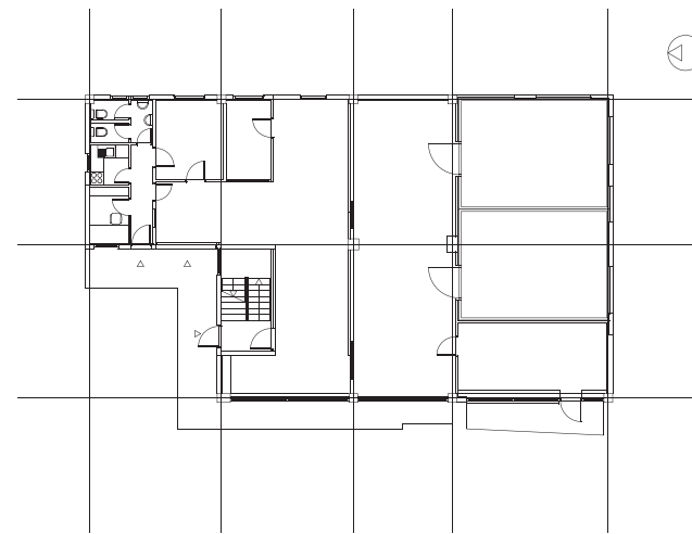
OSNOVA PRIZEMLJA
