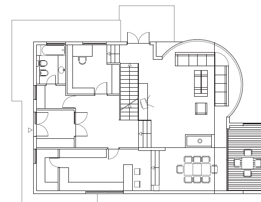
OSNOVA PRIZEMLJA
