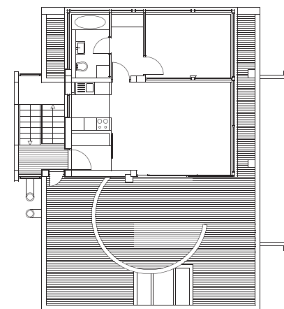
OSNOVA POTKROVLJA
