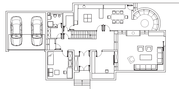
OSNOVA PRIZEMLJA
