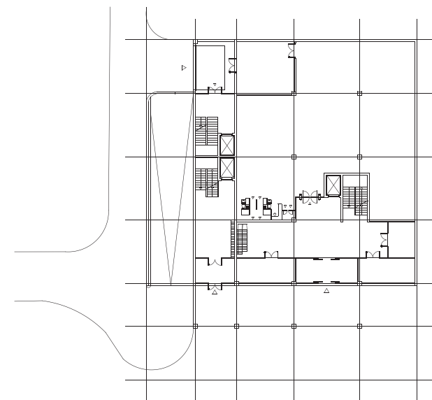
OSNOVA PRIZEMLJA
