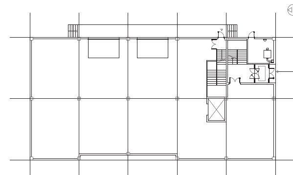
OSNOVA PRIZEMLJA
