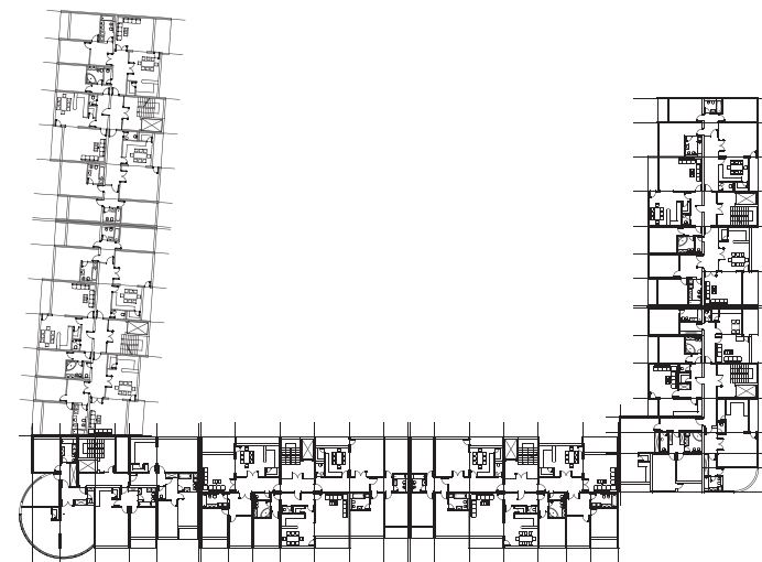
OSNOVA KARAKTERISTIČNE ETAŽE STAMBENOG DIJELA
