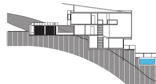
PRESJEK
